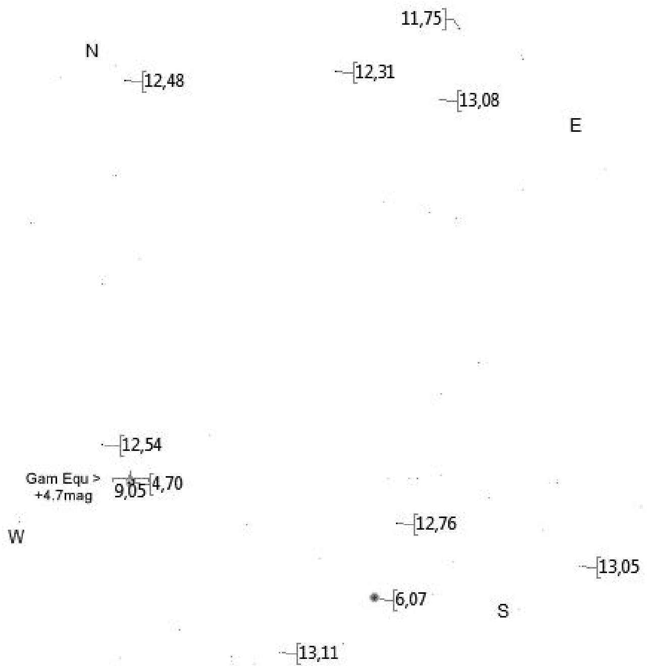
TML Gam Equ per Mitte Oktober 15' FoV
