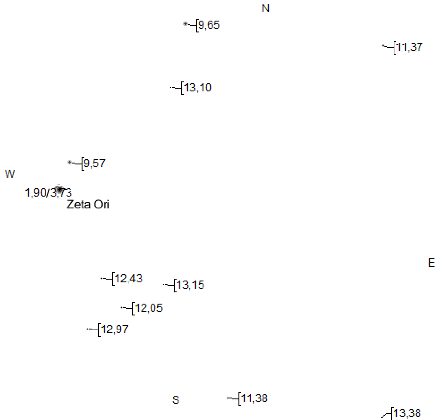
TML Zeta Ori per Mitte Jänner 15' FoV
